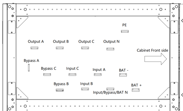
Рисунок 3.12. Соединительные клеммы отсека силовых модулей
