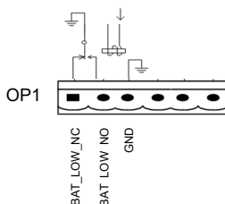
Рисунок 3.18. Схема интерфейса выходного релейного контакта предупреждения о низком напряжении АКБ
