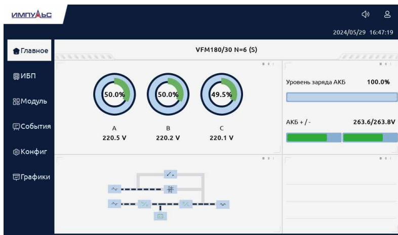
Рисунок 4.2. Главная страница
