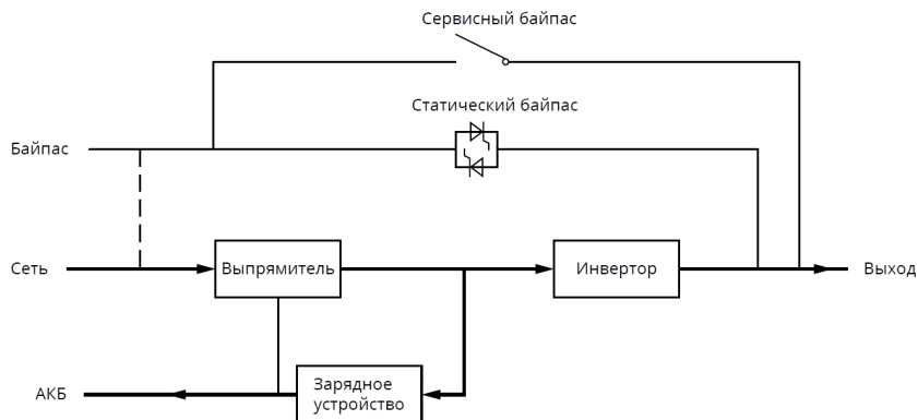
Рисунок 2.3. Функциональная схема нормального режима работы
