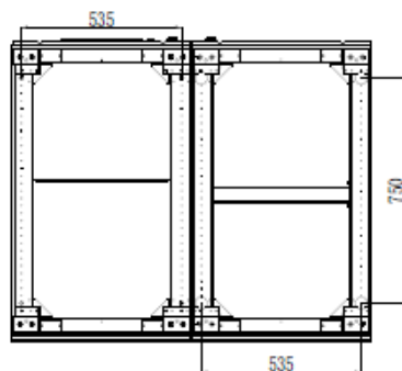
(б) Габариты шкафа на 8 слотов (конфигурация с выключателями)
