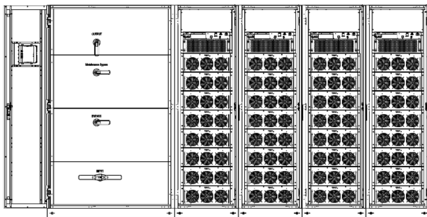
(и) Вид шкафа на 32 слота с открытой дверью
