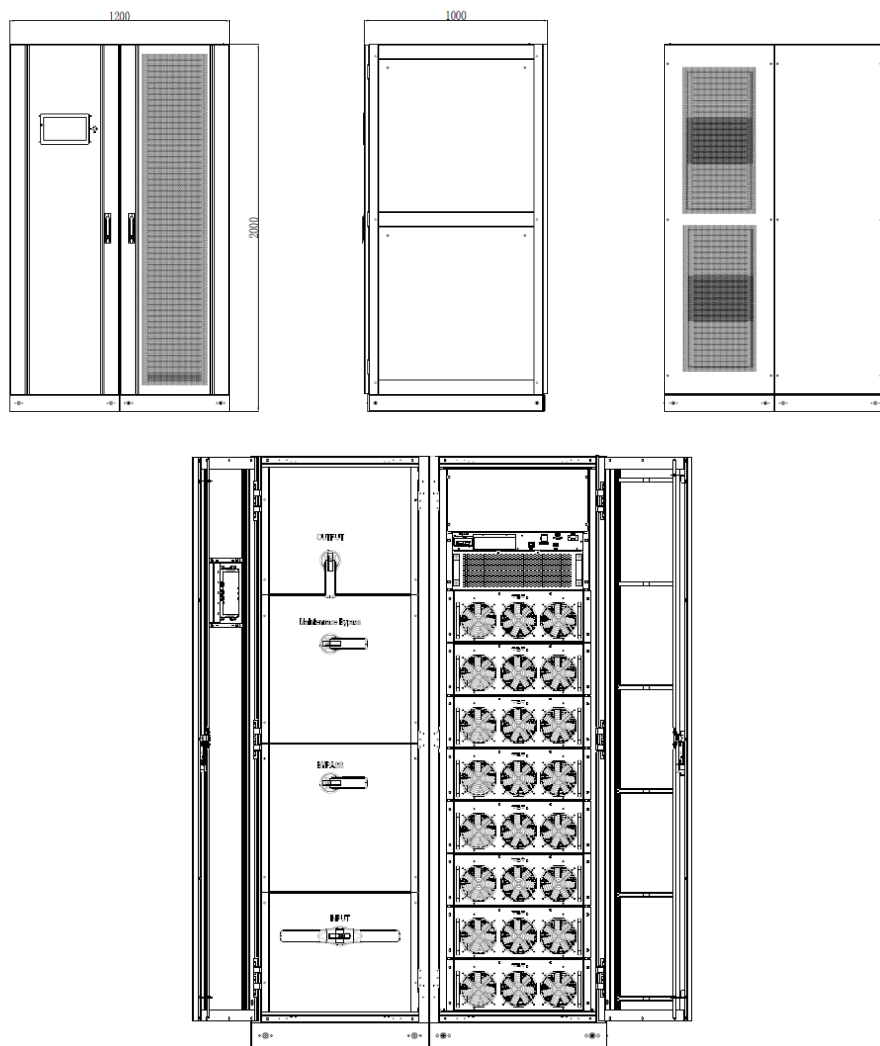
(б) Внешний вид шкафа на 8 слотов (конфигурация с выключателями, вид спереди и сзади, вид с открытой дверью)
