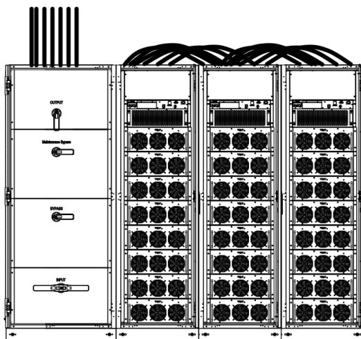
(в) схема кабельного ввода сверху в шкаф на 24 слота
