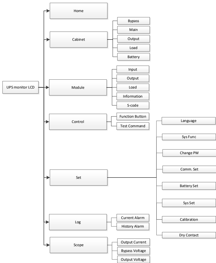
Рисунок 4.3. Схема структуры меню
