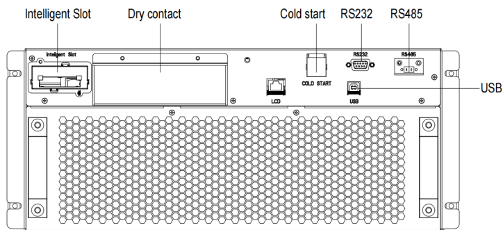
Рисунок 3.13. Схема интерфейсов обмена данными
