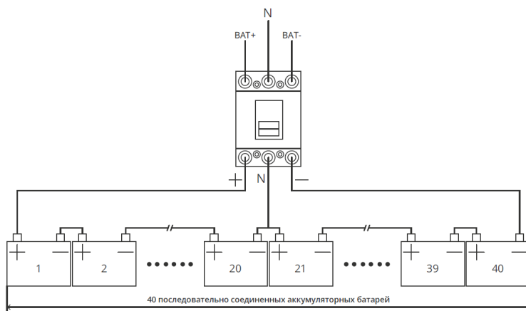
Рисунок 3.10. Схема соединения 12 В АКБ в массиве
