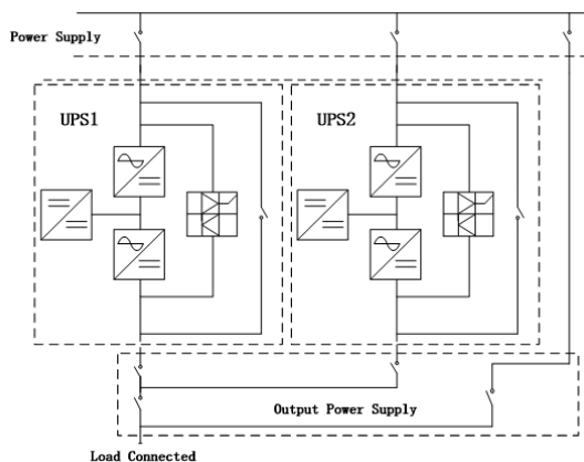
Рисунок 5.4. Схема параллельного подключения
