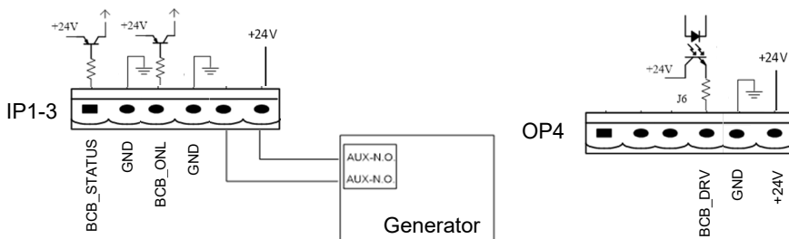
Рисунок 3.17. Порт АВ АКБ
