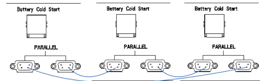
Рисунок 5.6. Схема параллельного подключения
