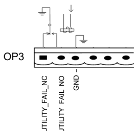
Рисунок 3.20. Схема интерфейса выходного релейного контакта предупреждения отказа сети
