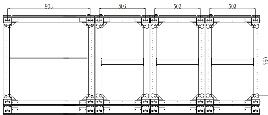
(в) Шкаф на 24 слота
