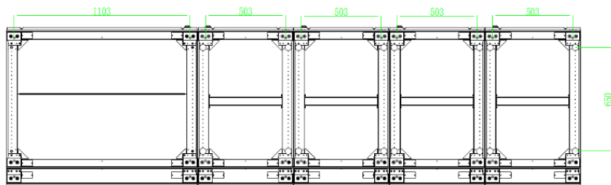
(г) Шкаф на 32 слота
