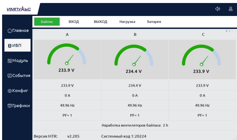
Рисунок 4.5. Меню шкафа
