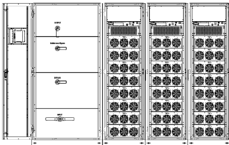
(е) Вид шкафа на 24 слота с открытой дверью
