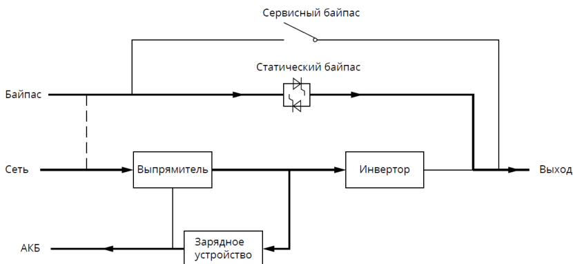
Рисунок 2.7. Схема экономичного режима
