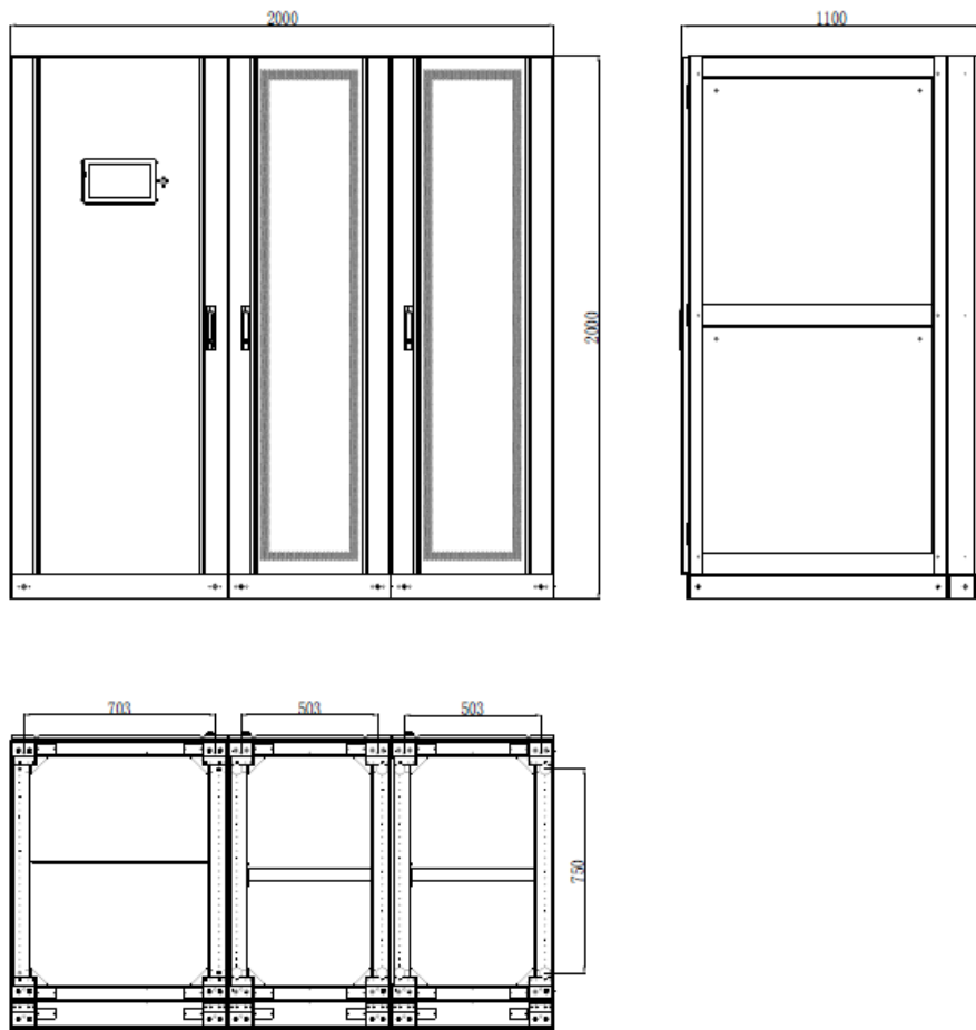
(в) Габариты шкафа на 16 слотов
