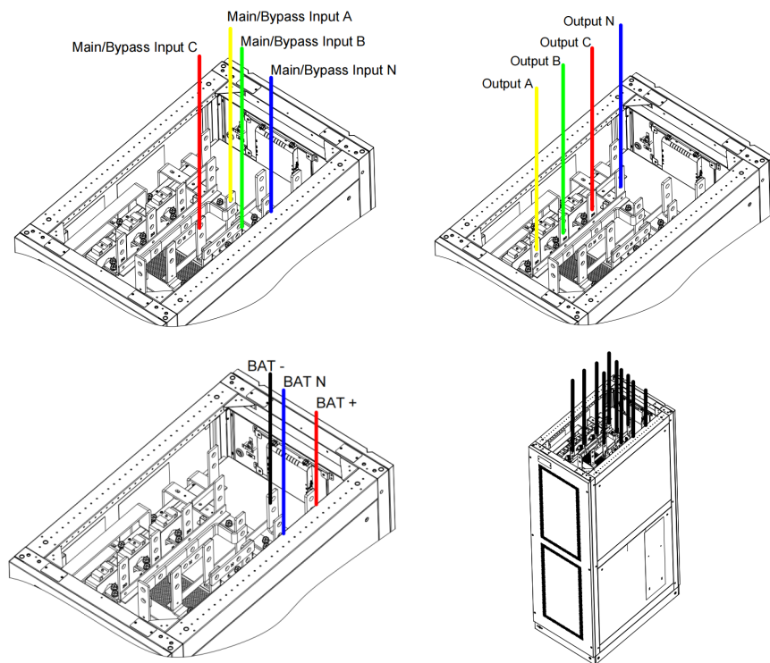
(а) схема кабельного ввода сверху в шкаф на 8 слотов (конфигурация без выключателей)
