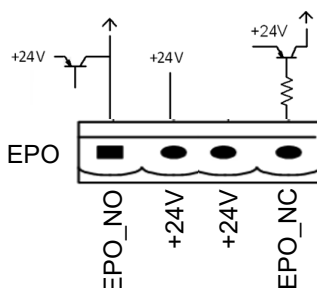
Рисунок 3.14. Схема входного порта для дистанционной подачи команды ЕРО
