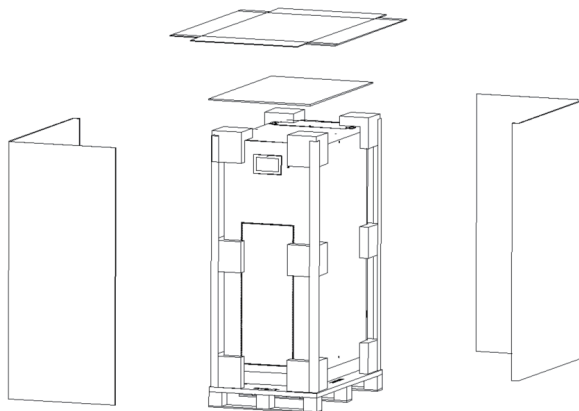
Рисунок 3.4. Разборка ящика
