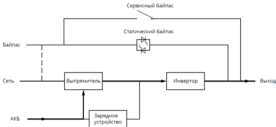
Рисунок 2.4. Схема режима работы от АКБ
