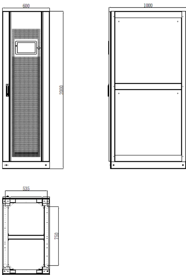
(а) Габариты шкафа на 8 слотов (конфигурация без выключателей)
