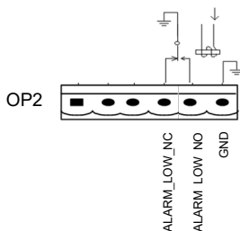
Рисунок 3.19. Схема интерфейса выходного релейного контакта общей тревоги
