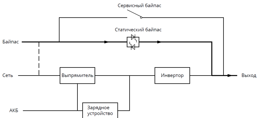
Рисунок 2.5. Функциональная схема режима байпаса
