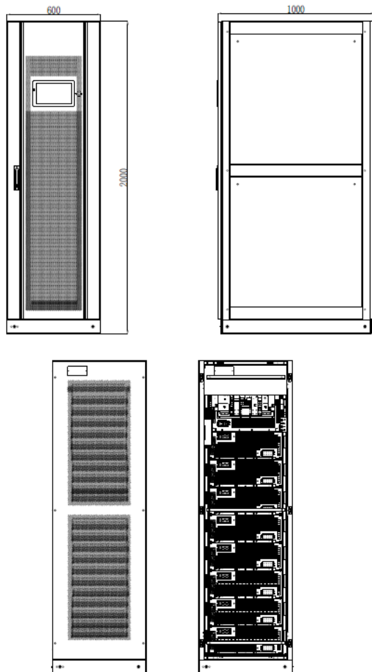
(а) Внешний вид шкафа на 8 слотов (конфигурация без выключателей, вид спереди и сзади, вид с открытой дверью)
