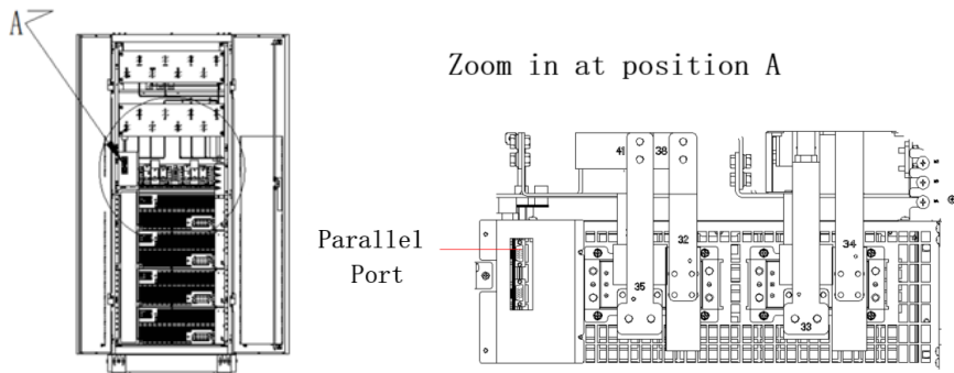
Рисунок 5.5. Расположение порта параллельного подключения ИБП
