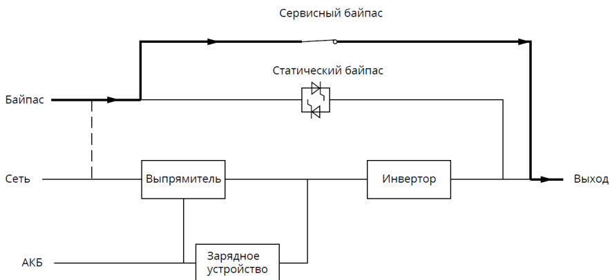
Рисунок 2.6. Функциональная схема режима сервисного байпаса
