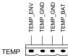
Рисунок 3.15. Порты TEMP 1-4 для определения температуры
