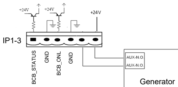
Рисунок 3.16. Схема входного порта для входа генератора
