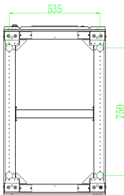
(а) Шкаф на 8 слотов (конфигурация без выключателей)
