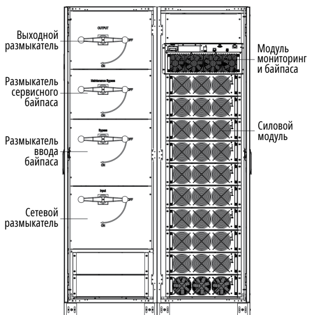
(в) Вид спереди шкафа с 10 слотами
