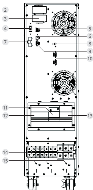
Рис. 4. ИБП 30-40 кВА Вид сзади (блок выводов без крышки)
