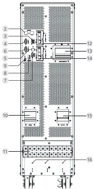
Рис. 3. ИБП 10-20 кВА Вид сзади (блок выводов без крышки)
