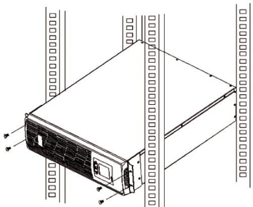
Рис. 3.2.3.4. Установка в стойку
