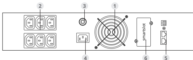
Рис. 2.3.2. Задняя панель ИБП в стойку (ЮНИОР ПРО РТ) 1000 ВА 2U
