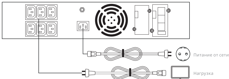
Рис. 3.2.3.1. Схема подсоединения входа/выхода стойки ЮНИОР ПРО РТ 24V пост. тока
