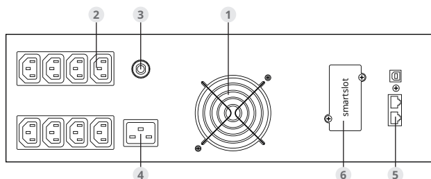
Рис. 2.3.2. Задняя панель ИБП в стойку (ЮНИОР ПРО РТ) 2000 - 3000 ВА 3U
