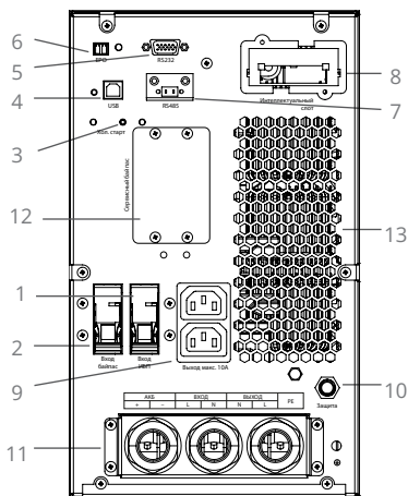
Рисунок 2.3. Вид сзади (ФОРА Н 6000/10000)
