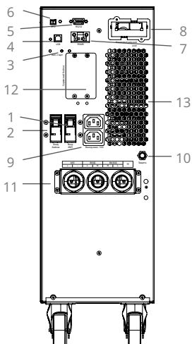
Рисунок 2.4. Вид сзади (ФОРА 6000/10000)
