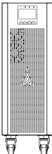
Рисунок 2.2. Вид спереди (версия со встроенными АКБ)
