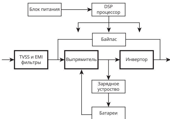
Рисунок 2.5. Система ИБП
